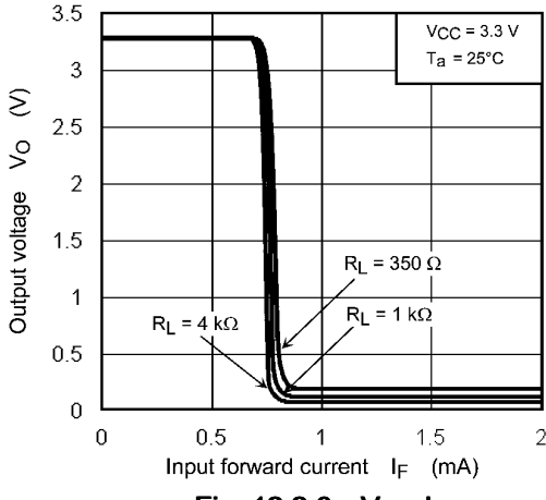
Fig. 12.2.6 V_O - I_F
