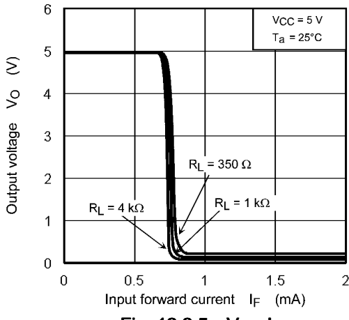
Fig. 12.2.5 V_O - I_F
